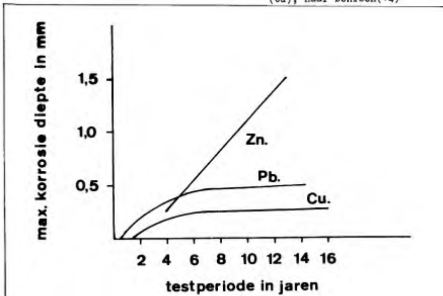
fig. 3 De max. korrosiediepte in de bodem t.o.v. de tijd van Zink (Zn), Lood (Pb) en Koper (Cu), naar Denison (14)
