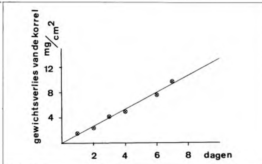
fig. 2 Het korrosiegedrag van een 3,3mm loodkorrel in een gesimuleerde kunstmaag, naar Kimball en Munir, 1971 (au) (1mg=0,001 gram)
